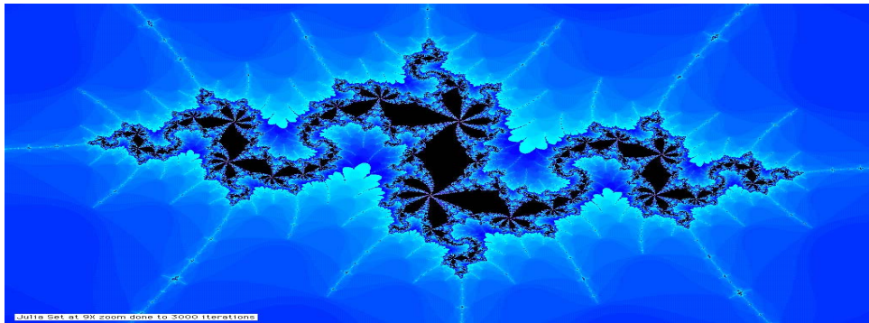
Figura 1 – Fractal produzido pelo computador
